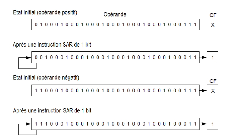
fonctionnement de l'instruction SAR 7
