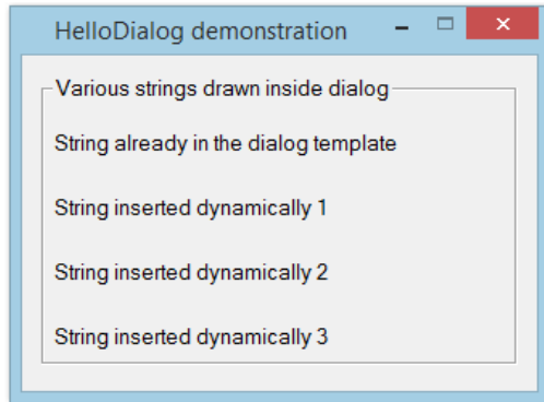
fig. 1 – première fenêtre
